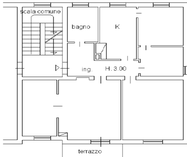
PIANO PRIMO
